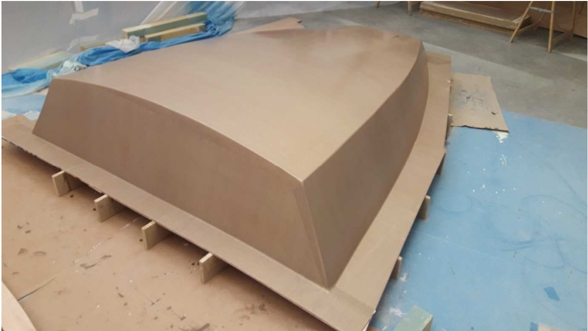
ROOF de FLOW 19 : Sandwich bambou / verre / mousse PET / epoxy
